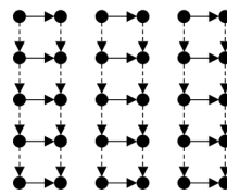
Fig. 1. Sparse grid
