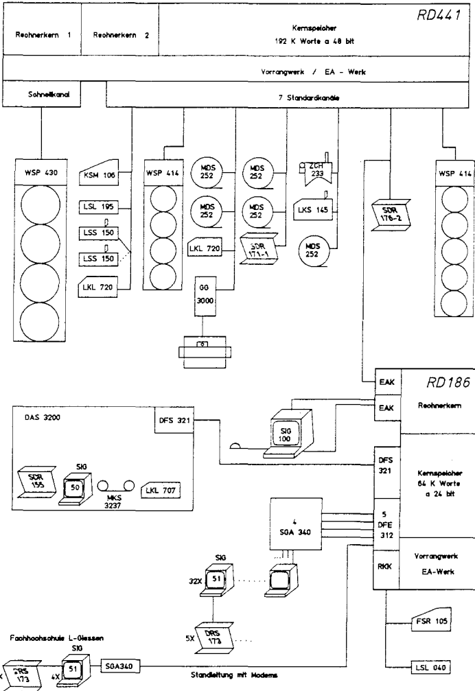
Abb. 2: Diese Übersicht über das Teilnehmer-Rechensystem TR 440 wurde mit dem Zeichengerät Geograph 3000 Aristomat hergestellt.
