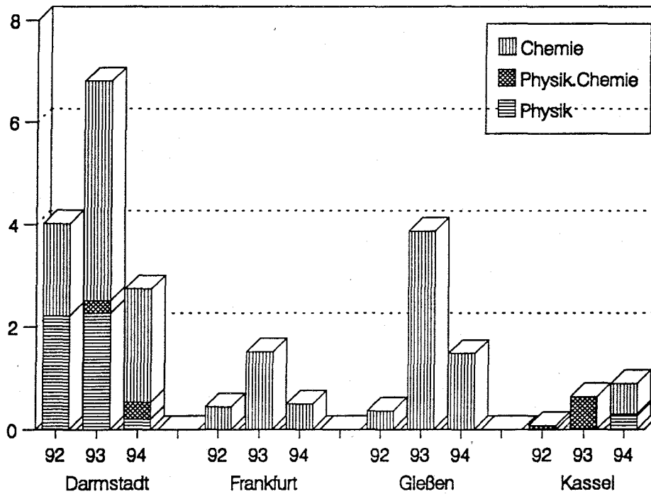
CPU-Stunden (Tausend)
