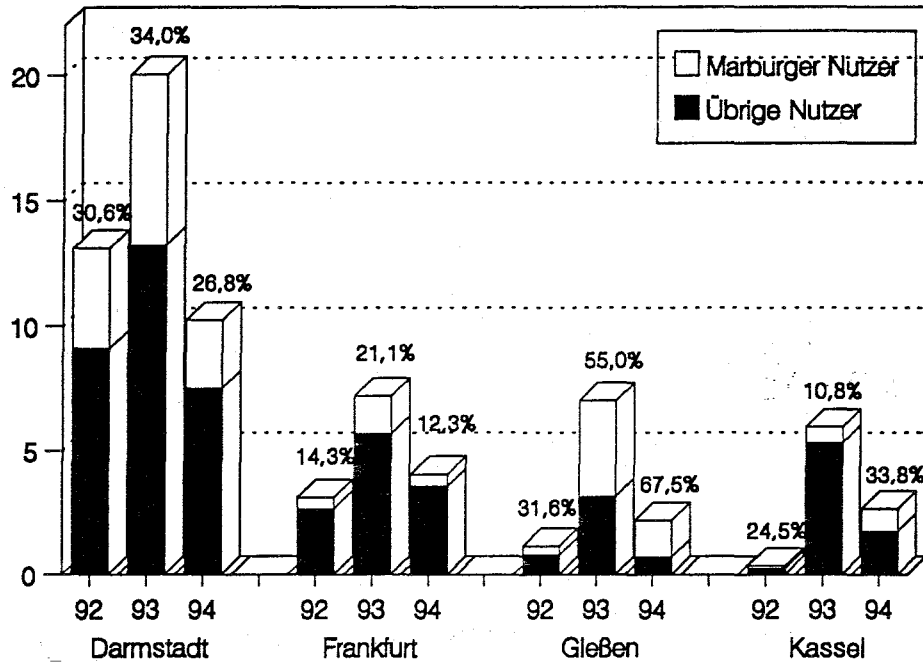
CPU-Stunden (Tausend)
